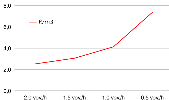
Evolution du coût d'épandage en fonction de la vitesse de rotation des tonnes à lisier
