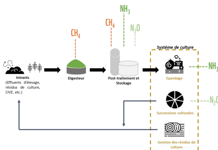
Figure 6. Impact des stratégies de post-traitement des digestats sur les émissions gazeuses à l'échelle de la filière (D'après Girault et al. 2017)
